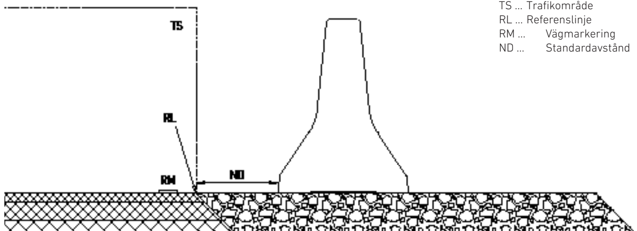
Bild 4 | Referenslinje.
