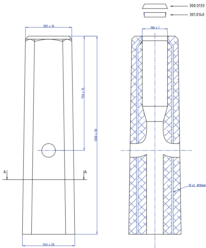
Snitt A-A
